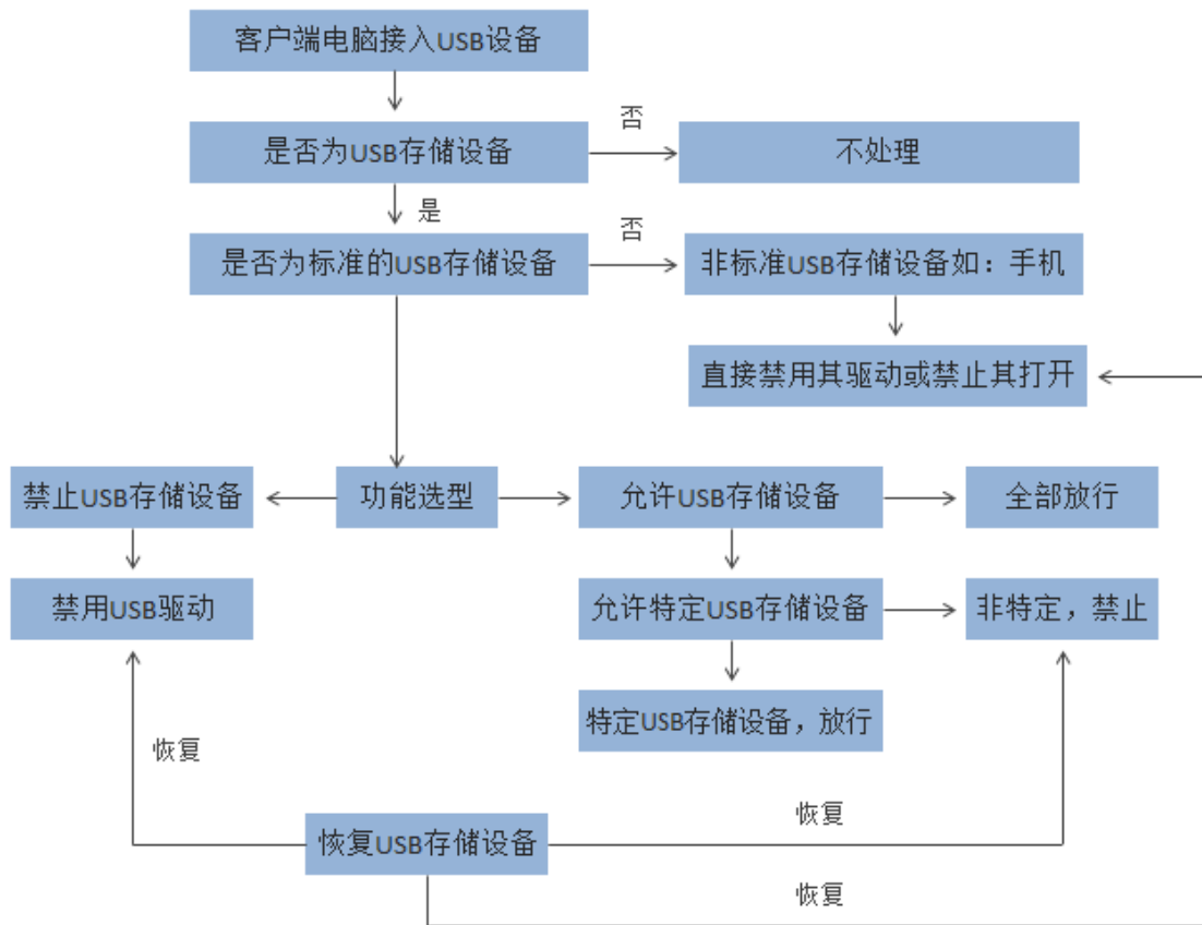
（图：USB 存储设备控制原理图）
